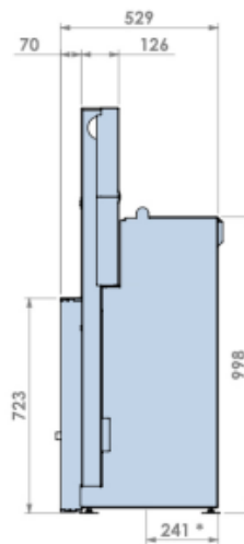
Zijaanzicht
