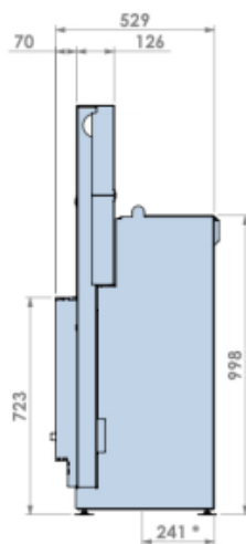
Zijaanzicht
