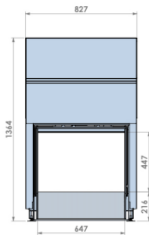
Vooranzicht
