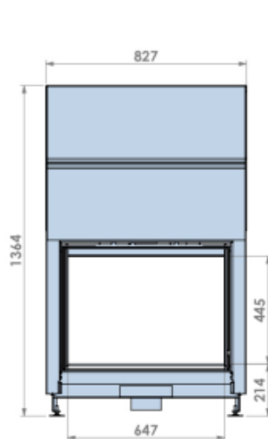
Vooranzicht
