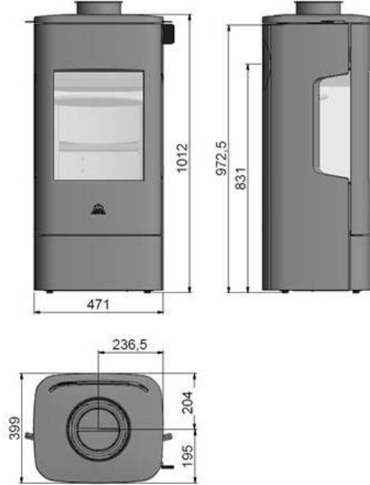
Jøtul F 233
