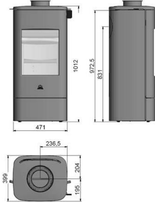
Jøtul F 232
