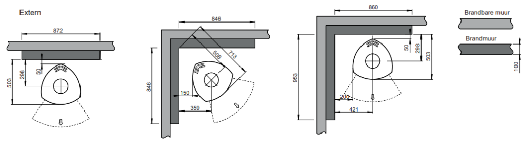
Jetul F 360 Advance Minimale afstand tot brandmuur
