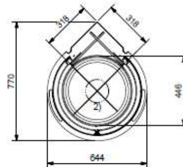
A-A ( 1 : 20 )
