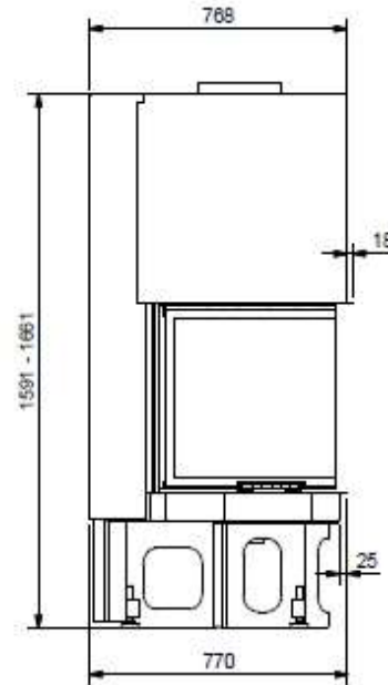
Grundriss Feuerstelle / Coupe sur foyer Sezione al piano fuoco / Layout fireplace
