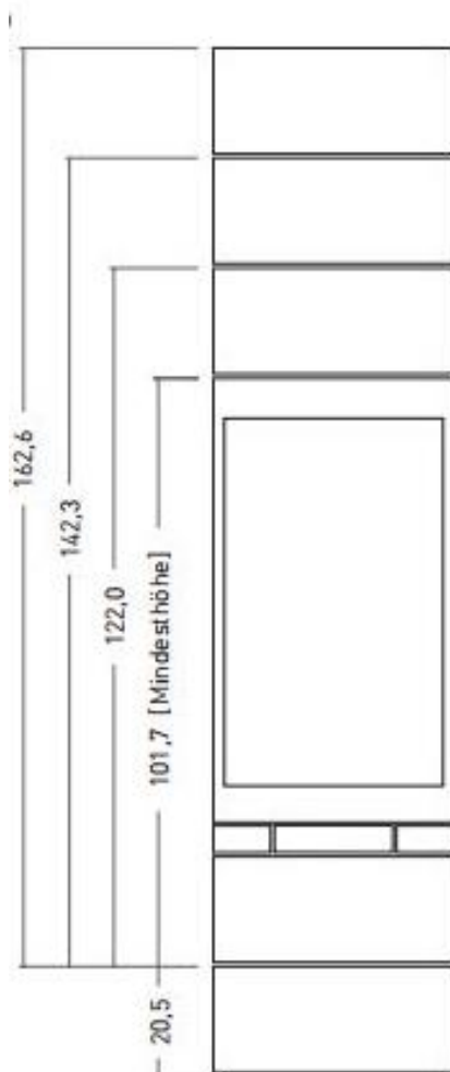
Frontansicht
