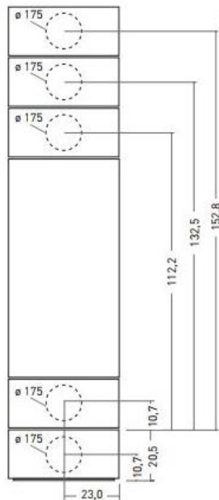
Rückansicht
