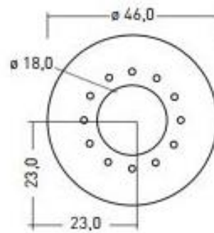
Frischluftzufuhr (unten)
