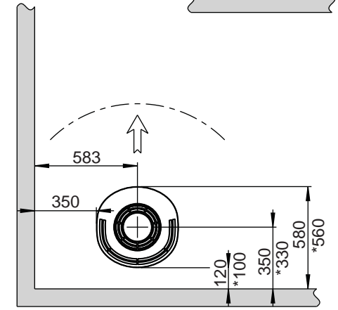
Brandbare muur
